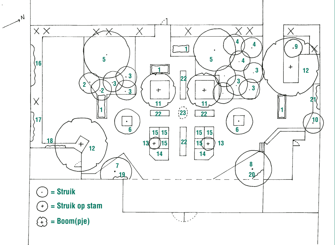
KAART 2 : Ontwerpplan voor de speelplaats.
